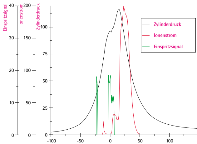
Ionenstromkurve
